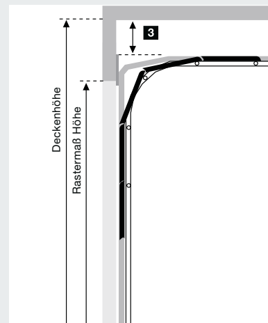
3 Freiraum für Garagen-Sectionaltore
