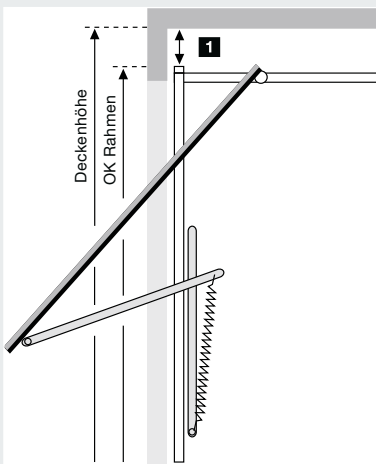
1 Freiraum für Berry-Schwingtore
