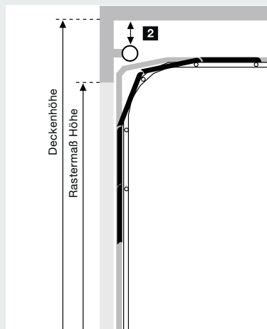
2 Freiraum für Garagen-Sectionaltore
